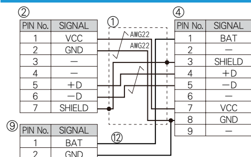
编码器（ABS）750W以下/1kW(仅限MX951) 固定电缆
