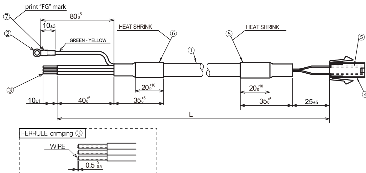
电机 750W以下/1kW (仅限MX951) 可动电缆
