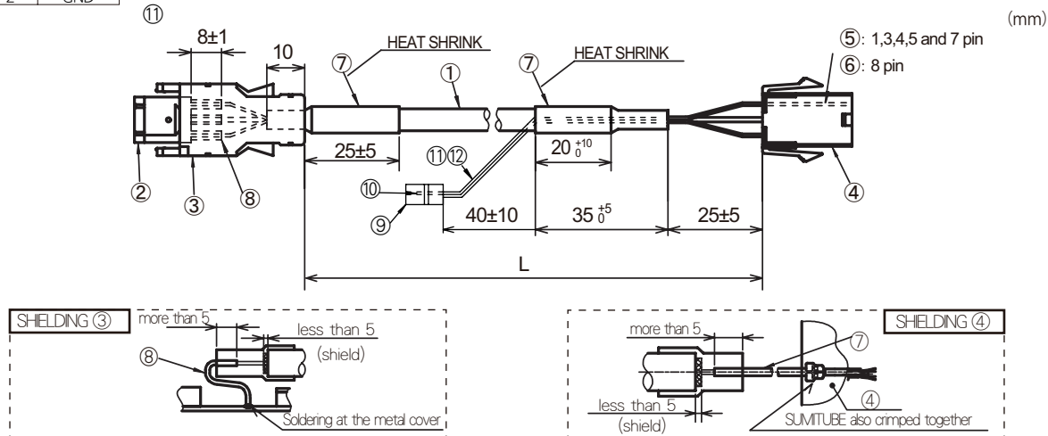
编码器（ABS）750W以下/1kW(仅限MX951) 可动电缆
